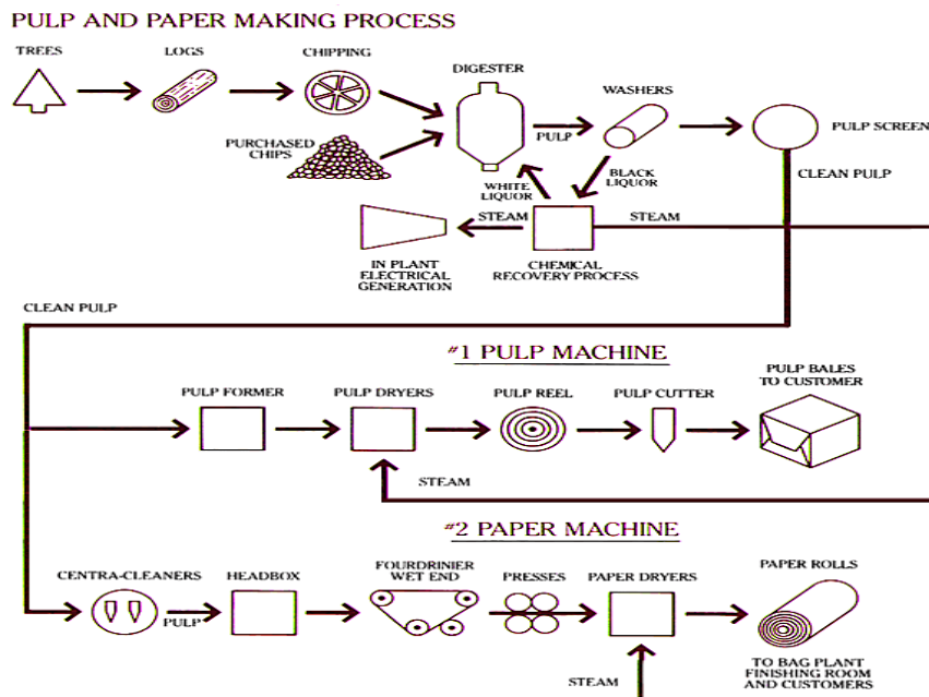
Gambar 2. Proses Produksi Kertas
