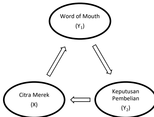
Gambar 1. Diagram Hasil Analisis Path Variabel Citra Merek, Word of Mouth dan Keputusan Pembelian.
